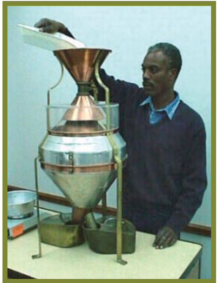
Boerner Divider
